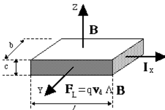
Geometria dell'effetto Hall
