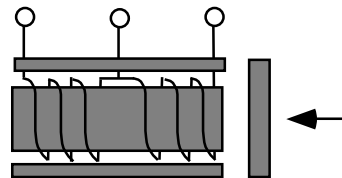
Sensore a riluttanza con nucleo fisso
